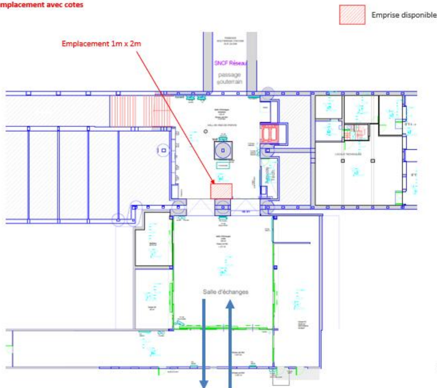
BESANCON VIOTTE Plan de l'emplacement avec cotes
